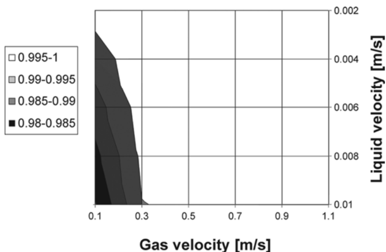
Linie konstantní relativní rychlosti disipace energie při synchronizovaných pulzacích kapalinou a plynem v systému toluen/voda - vzduch
