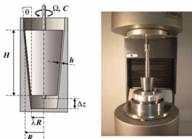
Originální KK sensor pro AWS viskozimetrii
