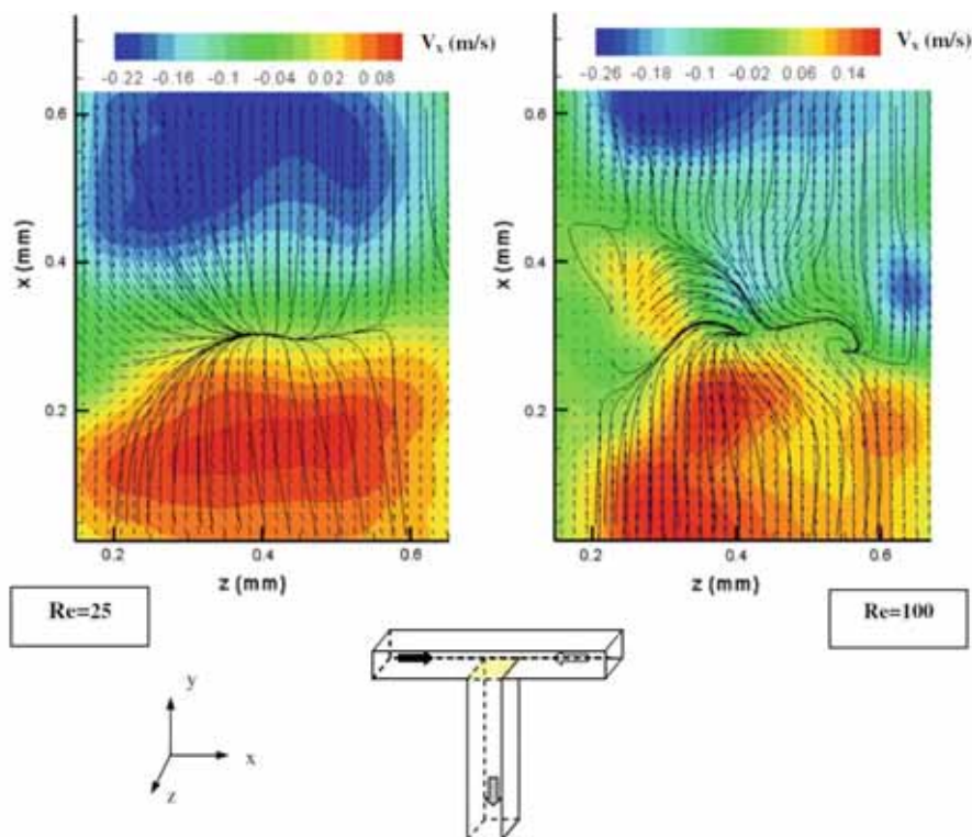
Rychlostní pole, proudnice a rychlostní profil v_x v mikromísíčovém tvaru T pro Re = 25 a Re = 100
