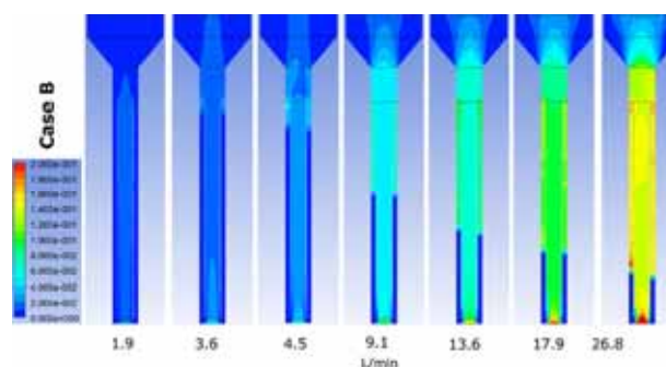
Barevná mapa lokální zádrže plynu (obj. zlomek plynné fáze) v „airlift“ reaktoru pro různé průtoky plynu na vstupu
