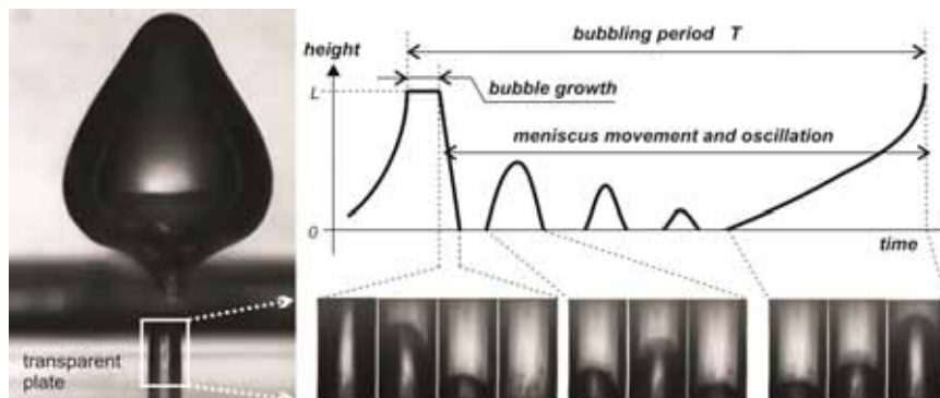
Studovaný klíčový jev – oscilace menisku – ovlivňující variabilitu velikosti bublin a synchronnost vzniku bublin na otvorech
