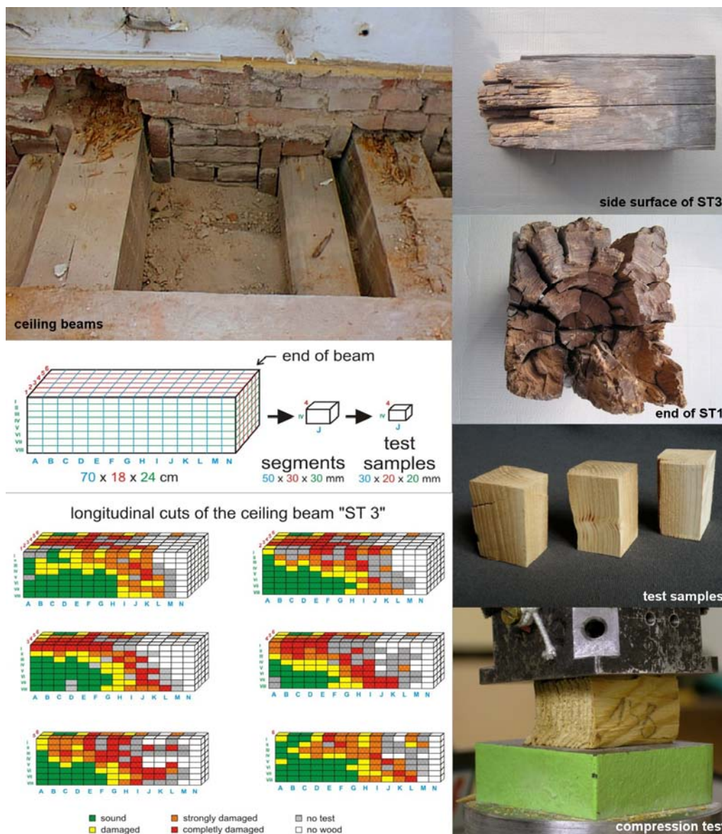
Degrační profil dřevěného konstrukčního prvku.
