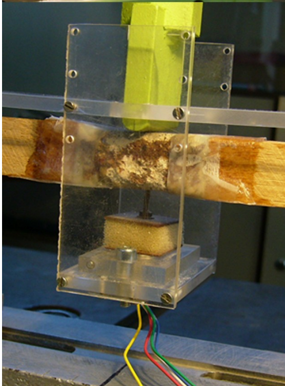
Uspořádání experimentu
