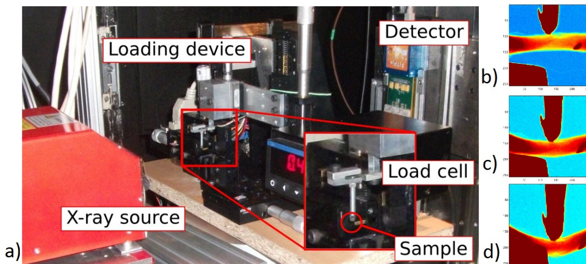
Mikrorentgenografické zobrazování deformací ve vzorku jednotlivé trabekuly namáhané třibodovým ohybem
