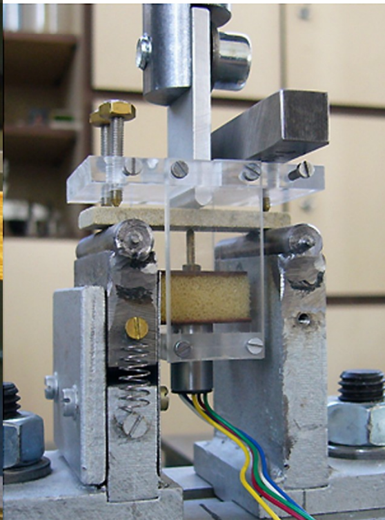
Uspořádání experimentu
