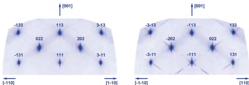
■ Obr. 5 Řezy reciprokým prostorem naměřených intenzitních map. Svislé stopy v okolí difrakčních maxim kolmé na povrch vzorku jsou důsledkem konečné tloušťky ozářeného objemu vzorku. Šikmé stopy difúzního rozptylu ve směrech [111] a [1\bar{1}\bar{1}] jsou způsobeny rozptylem záření na vrstevných chybách v rovinách (111) a (1\bar{1}\bar{1}) .
