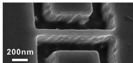
■ Obr. 3 Feromagnetická rezonance v nanosoučástce vyvolaná proudem a spin-orbitální interakcí [3].
