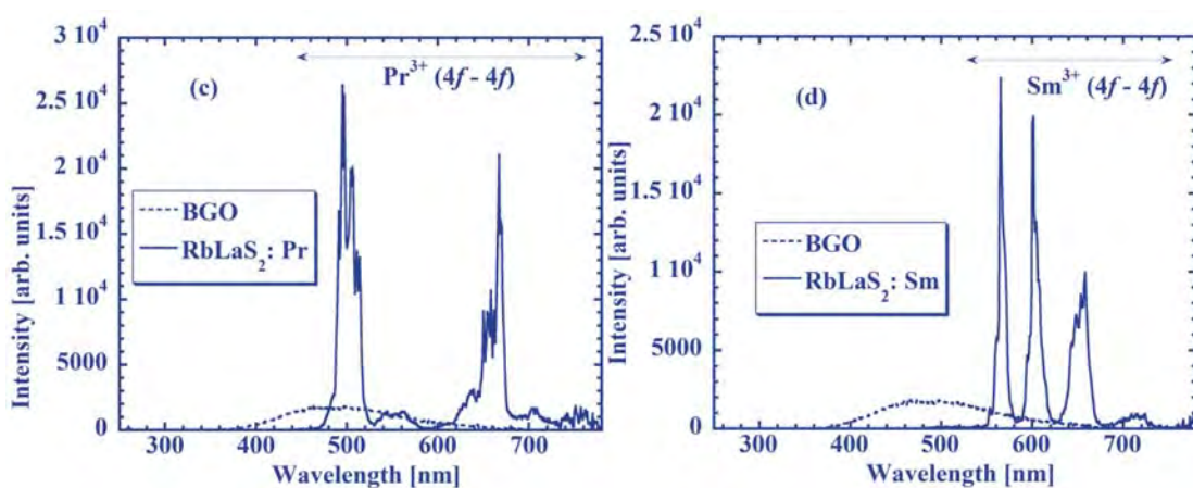
■ Obr. 17 Radioluminiscenční spektra sloučenin \text{RbLaS}_2:\text{Pr} a \text{RbLaS}_2:\text{Sm}
