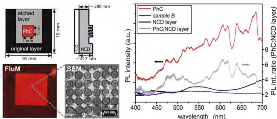
■ Obr. 14 Schématické znázornění fotonického krystalu z nanokrystalického diamantu, mikroskopický obrázek luminiscence krystalu v červené spektrální oblasti, detailní struktura krystalu z elektronového mikroskopu a spektrum luminiscence krystalu ukazující významné zesílení luminiscence v široké spektrální oblasti [28].
