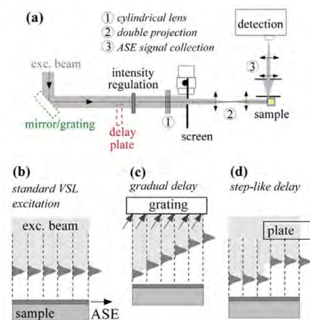
■ Obr. 12 Metoda VSL: (a) Obecné schéma experimentálního uspořádání. (b) Detail standardní metody VSL vhodné pro stacionární čerpání ve srovnání s naší modifikací metody dosahované (c) postupným zpožďováním budících pulzů optickou mřížkou nebo (d) stupňovitým zpožděním pulzů pomocí křemenné destičky.
