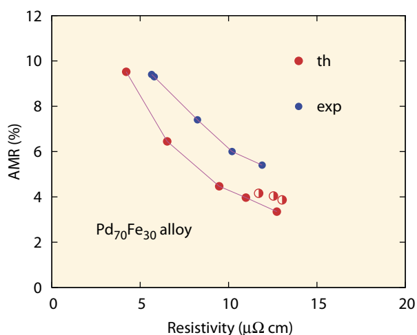
Obr. 1 Porovnání vypočteného poklesu anomální magnetoresistence při rostoucí neuspořádanosti s experimentálními daty. Výsledky pro částečně uspořádanou slitinu fcc \text{Pd}_{70}\text{Fe}_{30} (plné symboly), poloprázdné symboly odpovídají zcela neuspořádané slitině. Je zřejmé, že experimentu odpovídá částečně uspořádaná slitina, nikoliv neuspořádaná fáze, protože její vypočtená resistivita není nikdy menší než 10 \mu\Omega\text{cm} .
