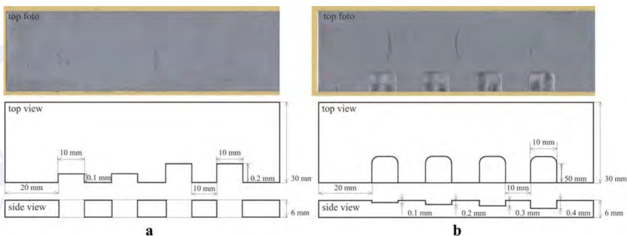
■ Obr. 13 Vzorky pro modelování defektů na tupých svarech z oceli AISI 304
