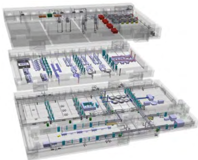
■ Obr. 9 Schéma rozmístění technologického zázemí (horní podlaží), laserového zařízení (přízemí) a experimentálních pracovišť (podzemní podlaží) v budově ELI.
