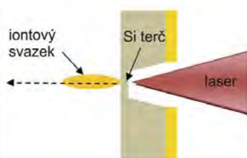
■ Obr. 2 Porovnání TOF signálů iontových kolektorů, z nichž jeden byl stíněn 8 \mu\text{m} Al fólií, která absorbovala XUV záření emitované plazmatem generovaným laserovým svazkem o intenzitě 2 \times 10^{16} \text{ W/cm}^2 . Iontový svazek byl emitován ze zadní strany hydrogenovaného 17 \mu\text{m} tenkého Si terče.
