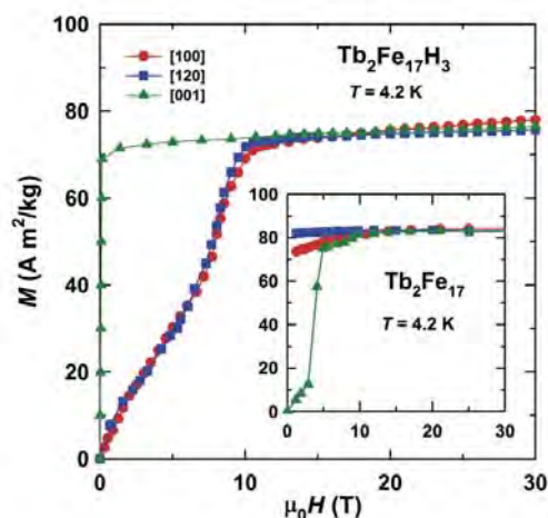
■ Obr. 8 Magnetizační křivky podél hlavních krystalografických os měřené při 4,2 K na monokrystalu hydridu \text{Tb}_2\text{Fe}_{17}\text{H}_3 v porovnání s \text{Tb}_2\text{Fe}_{17} (vložený panel). Je patrné, že osa [001] je v mateřské sloučenině nesnadnou osou, avšak v hydridu se stává osou snadnou.
