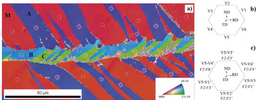
■ Obr. 9 Struktura monokrystalu hořčíku po deformaci válcováním zviditelněná difrakcí zpětně odražených elektronů (EBSD). Pomocí šestibokých hranolů je naznačena orientace jednotlivých dvojčat. V původní matici M jsou primární dvojčata A a B, uvnitř těchto dvojčat pak sekundární („zelená“) dvojčata C – všechny typu {10-12}.
