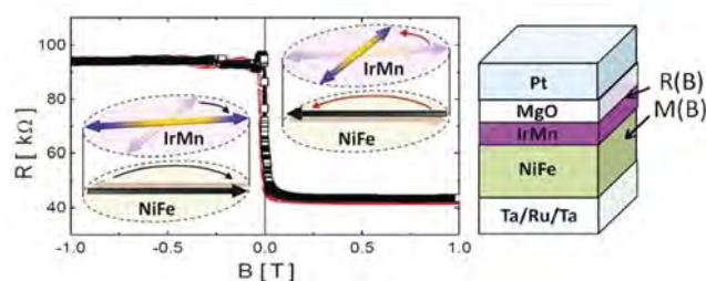
Antiferomagnetická tunelovací součástka (vpravo) a její magnetoresistenční signál
