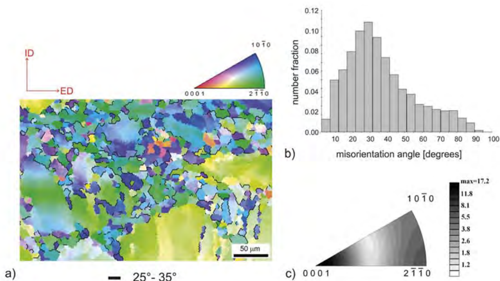
■ Obr. 10 Orientace zrn v hořčíku deformovaného metodou ECAP. (a) Hranice s natočením 30^\circ \pm 5^\circ jsou vyznačeny černě; (b) distribuce úhlu natočení zrn; (c) distribuce rotačních os pro natočení hranic 30^\circ \pm 5^\circ .
