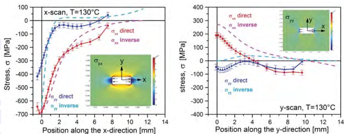
■ Obr. 15 Rozložení vnitřních pnutí v ocelové desce s úmyslně zabudovanými vměstkem ze slitiny NiTi zahřáté na teplotu 130^{\circ}\text{C} určené z neutronových difrakčních měření (neutron stress scanning) pomocí přímého výpočtu (direct) a inverzního FEM modelování (inverse).
