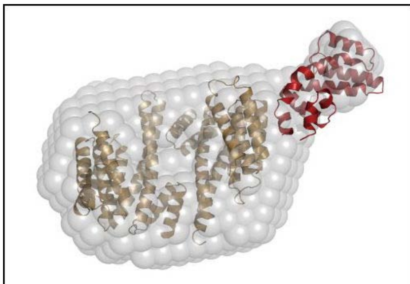
Obr. 3. Struktura komplexu 14-3-3 proteinu (světle hnědá) s regulátorem G-proteinové signalizace 3 (červená) navržená na základě SAXS (nízkoúhlový rozptyl rentgenového záření) měření. Molekulární obálka vypočtená ze SAXS dat je znázorněna šedě.
