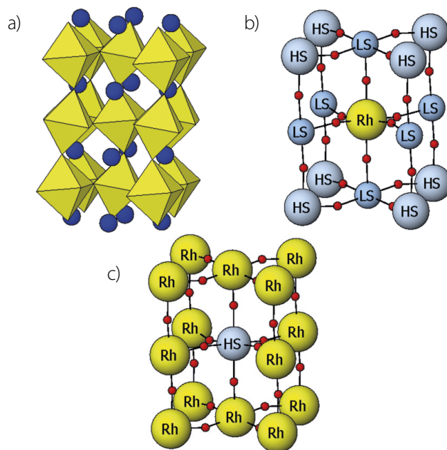
■ Obr. 6 a) Perovskitová struktura \text{LaCo}_{1-x}\text{Rh}_x\text{CrO}_3 s oktaedry \text{Co}_{1-x}\text{Rh}_x\text{O}_6 , b) lokální uspořádání \text{Rh}^{3+} a \text{Co}^{3+} v nízkém a vysokém spinu pro malé koncentrace Rh, c) lokální uspořádání \text{Rh}^{3+} a \text{Co}^{3+} ve vysokém spinu pro velké koncentrace Rh
