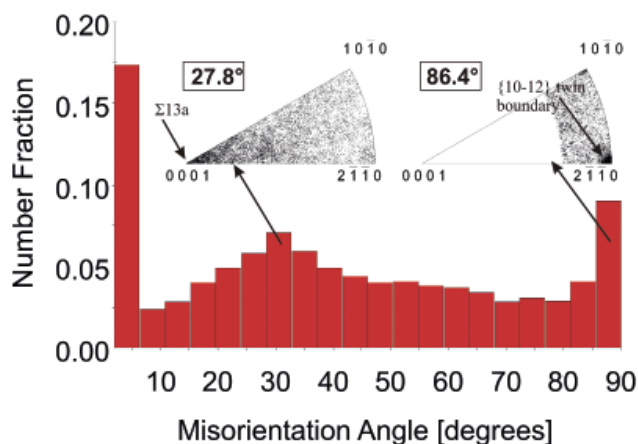
■ Obr. 7 Distribuce úhlů natočení (>2°) pro vzorek hořčíku po čtyřnásobném zpracování ECAP s protitlakem při pokojové teplotě. Dva píky odpovídají natočení 27,8° ( \Sigma 13 koincidenční hranice {10-12}) a 86,4° (dvojčatová hranice).
