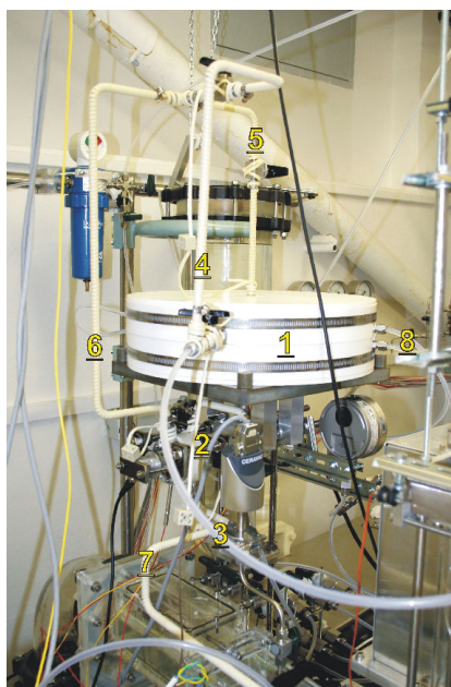
■ Obr. 6 Odparník molekulárního jódu v radiofrekvenční aparatuře, Ar výboj, komora-injektor
