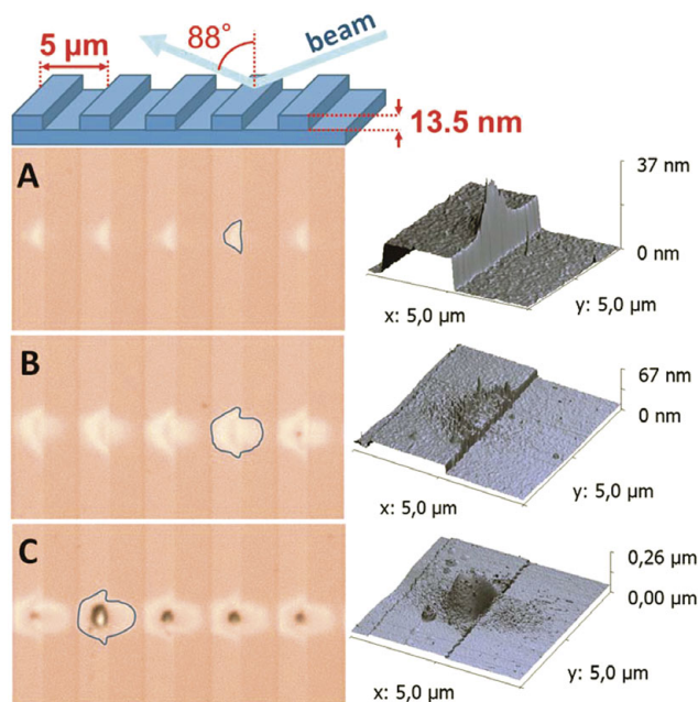
■ Obr. 12 Následky ozáření reflexní mřížky (strukturovaný kremíkový substrát byl magnetronově potažen 45 nm silnou vrstvou amorfního uhlíku; profil mřížky a podmínky jejího ozáření jsou znázorněny zcela nahoře) na fluencích 356 mJ/cm 2 (A), 806 mJ/cm 2 (B) a 1115 mJ/cm 2 (C) měkkého rentgenového laserového záření
