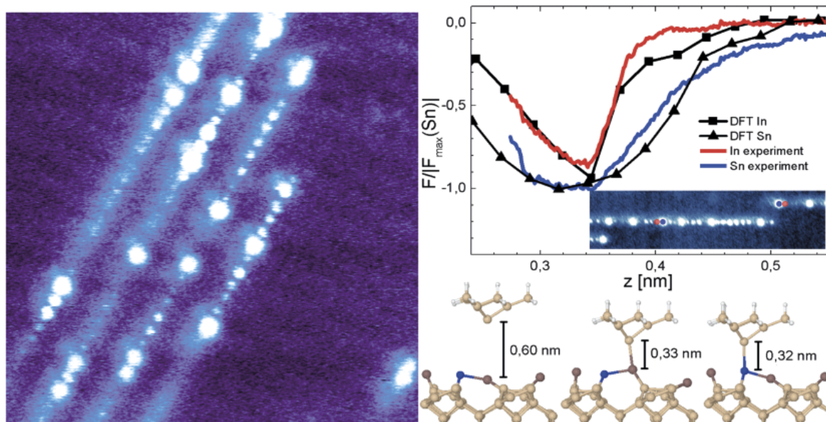
Obrázek řetízků Sn–In na povrchu Si(100) v atomárním rozlišení (vlevo), porovnání experimentálních a teoretických charakteristických silových křivek nad atomem Sn a In (uprostřed) a schematický obrázek teoretických výpočtů (vpravo)
