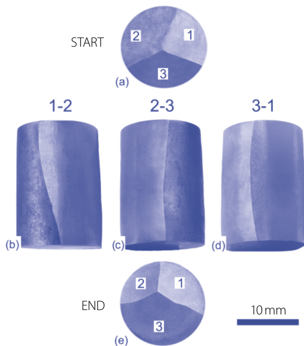
■ Obr. 8 Naleptaný trikrystal po růstu. a) kolmý řez na osu růstu v místě zárodku (START); b), c), d) boční povrchy s jednotlivými hranicemi 1–2, 2–3 a 3–1; e) kolmý řez na osu růstu na konci růstu (END).
