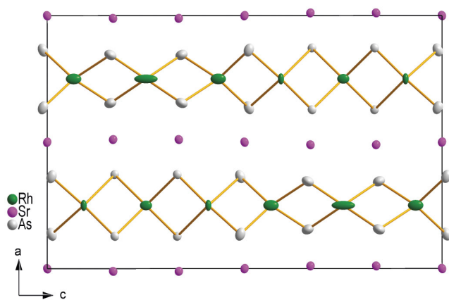
■ Obr. 4 Modulovaná struktura \beta\text{-SrRh}_2\text{As}_2 zobrazená v projekci podle krystalografické osy b . Elipsoidy výchylek atomů Rh vykazují výrazné modulace.
