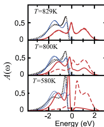
Elektronové spektrum \text{Sr}_2\text{IrO}_4 při různých teplotách. Otevření zakázaného pásu při 580 K souvisí s nástupem antiferomagnetického uspořádání.
