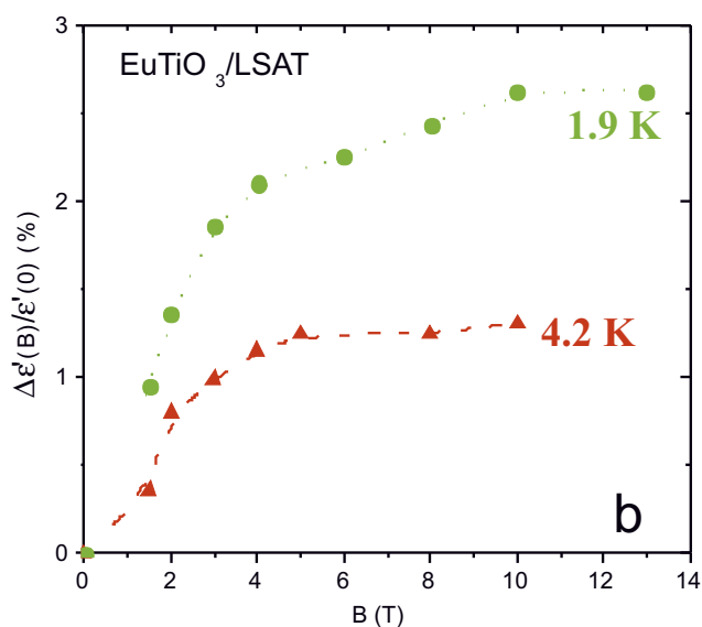
■ Obr. 4 a) Infračervená reflektance tenké vrstvy \text{EuTiO}_3 měřená při 1,9 K v závislosti na magnetickém poli: posuv fononové frekvence je jasně vidět. Vložený obrázek ukazuje nesouměřitelné reflexe (rovina 1/2kl) v elektronové difrakci monokrystalického \text{EuTiO}_3 při pokojové teplotě; b) závislost statické permitivity na magnetickém poli získaná z infračervených spektrů filmu \text{EuTiO}_3 naneseného na substrát LSAT.
