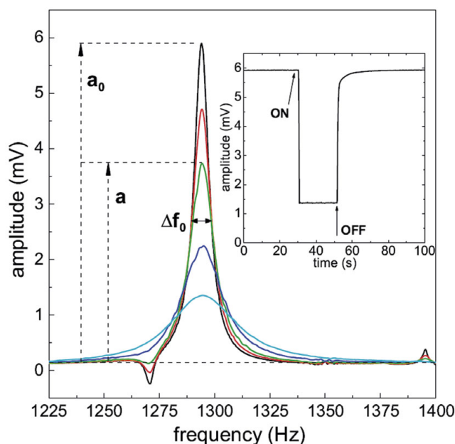
■ Obr. 6 Útlum rezonance druhého zvuku při rostoucí rychlosti proudění; ve vloženém obrázku: změna amplitudy druhého zvuku v čase, po zapnutí a vypnutí pohybu vlnovce
