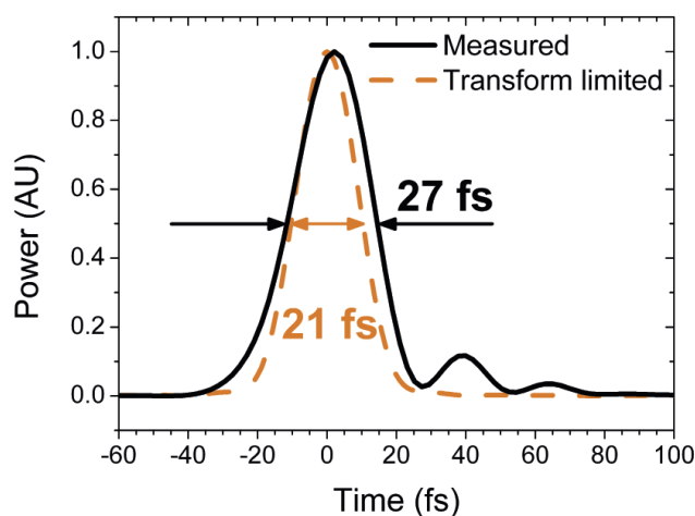
■ Obr. 3 Schéma laserového systému pro realizaci techniky OPCPA a změřený časový průběh zesíleného terawattového pulsu na vlnové délce 800 nm po zkrácení v optickém kompresoru
