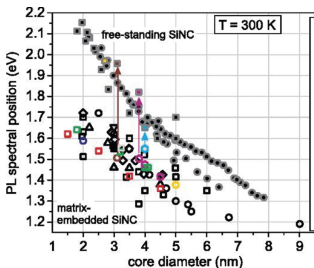
■ Obr. 9 Souhrn experimentů, ukazující energii fotonu maxima luminiscenčního pásu jako funkci velikosti oxidovaných Si nanokrystalů (NC). Symboly ohraničené šedí značí volné nanokrystaly, prázdné symboly označují nanokrystaly zabudované do matrice. Různé tvary symbolů značí různé metody
