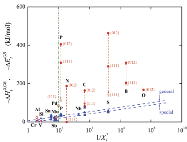
■ Obr. 3 Závislost energie, \Delta E_i^{GB} , a standardní entalpie, \Delta H_i^{0,GB} , segregace různých příměsí na hranicích zrn na reciproké rozpustnosti, X_i^* , při 800 K v \alpha -Fe. Trojúhelníky reprezentují experimentální hodnoty \Delta H_i^{0,GB} , kroužky jsou DFT hodnoty. Čárkované linie jsou predikované meze \Delta H_i^{0,GB} pro speciální a obecné hranice. Vertikální čerchovaná linie je rozpustnost 1 at.% při 800 K.
