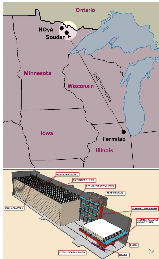
■ Obr. 2 Mapa na obrázku nahoře schematicky znázorňuje polohu laboratoře Fermilab a a vzdáleného detektoru NOvA. V dolní části je zobrazen cílový stav vzdáleného detektoru NOvA. V roce 2012 byla postavena čtvrtina detektoru – šrafovaná část vlevo.
