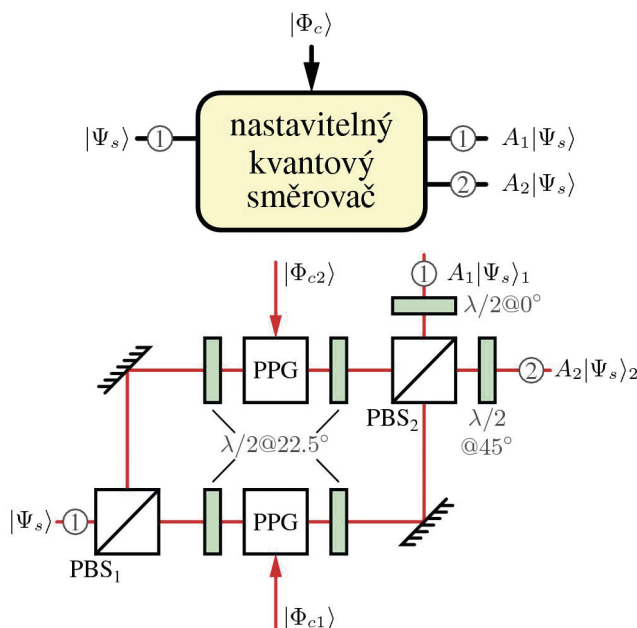
Obr. 1 Funkční schéma (nahore) a část lineárně optického návrhu (dole) kvantového směrovače. |\Psi_s\rangle a |\Phi_c\rangle značí signální a kontrolní kvantový stav, PPG programovatelnou změnu fáze a PBS polarizační dělič.
