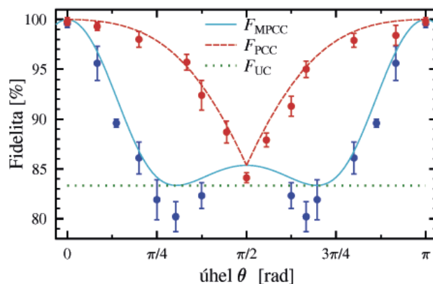
Obrázek vlevo – schéma experimentálního uspořádání. Vpravo – fidelita klonovaných stavů jako funkce úhlu distribuční funkce \theta pro tři význačné režimy: univerzální klonování (UC), fázově kovarianční klonování (PCC), zrcadlově fázově kovarianční klonování (MPCC). Čáry odpovídají teoretické předpovědi, značky představují měřené hodnoty.
