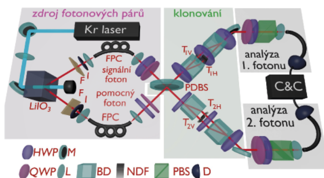
Obrázek vlevo – schéma experimentálního uspořádání. Vpravo – fidelita klonovaných stavů jako funkce úhlu distribuční funkce \theta pro tři význačné režimy: univerzální klonování (UC), fázově kovarianční klonování (PCC), zrcadlově fázově kovarianční klonování (MPCC). Čáry odpovídají teoretické předpovědi, značky představují měřené hodnoty.
