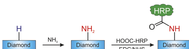
■ Obr. 12 Schematické zobrazení funkcionalizace povrchu nanokrystalické diamantové vrstvy amino skupinou a avidin-peroxidázou, tzv. karbodiimidovou metodou
