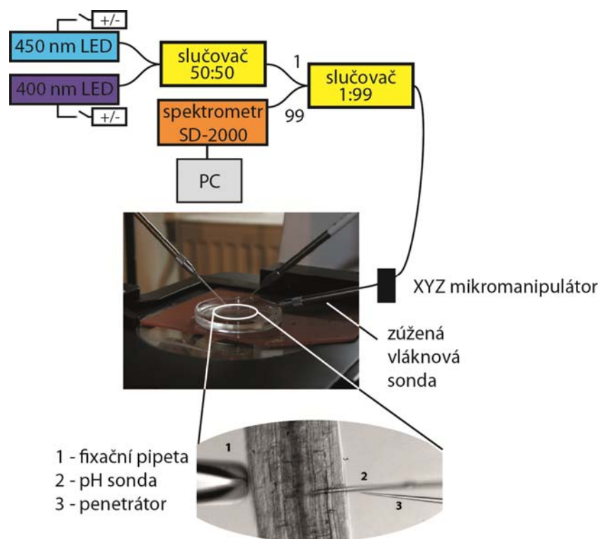
Obr. 1: Schéma měřicí aparatury (nahore), fotografie měřicího stanoviště s mikromanipulátorem (uprostřed) a mikroskopová fotografie se zavedenou sondou do kořínku huseníčku.
