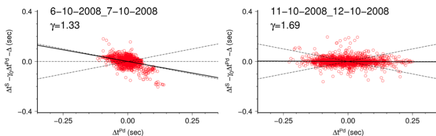
Dvojité difference časů příchodu S a P vln pro dva časové intervaly během seismického roje 2008, které se výrazně liší poměrem rychlostí \gamma = v_P/v_S .
