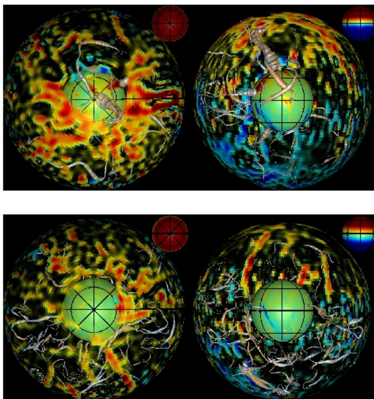
Model silného/slabého magnetické pole ve vnějším jádře Země se silným (nahore) a slabým (dole) polem v polární oblasti. Červené/žluté odstíny značí orientaci pole směrem ven a modré/zelené odstíny směrem dovnitř.
