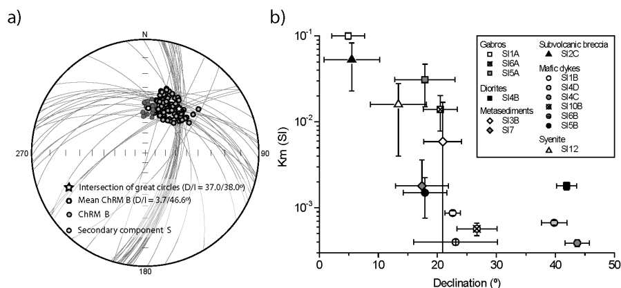
a) Stereografická projekce (spodní polokoule) charakteristické remanentní magnetizace. b) Graf ukazující vztah paleomagnetických deklinací a magnetické susceptibility ( K_m ) pro různé lokality/litologie masivu Sines.
