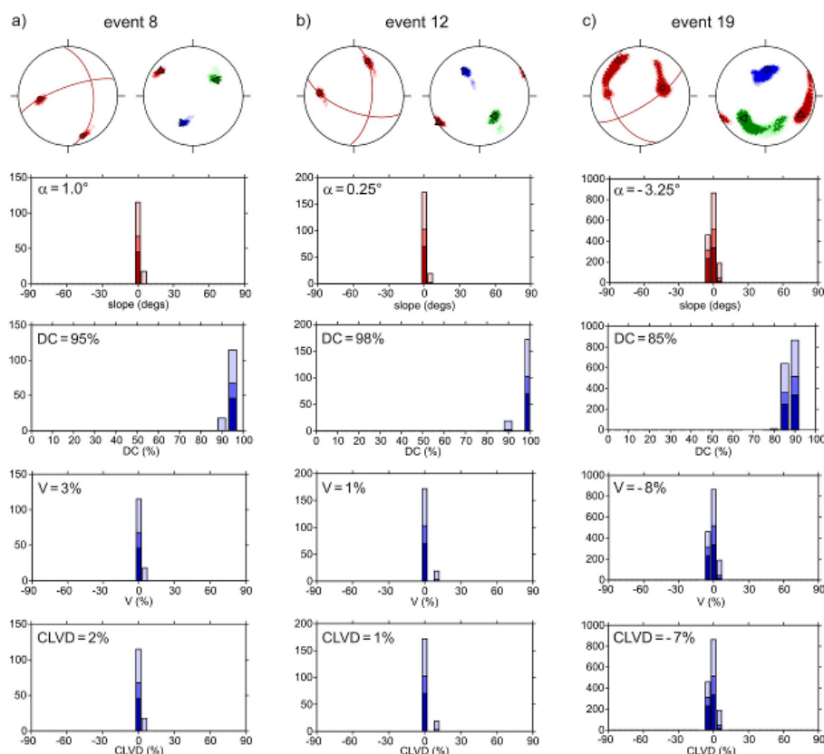
Srovnání momentového tenzoru (nahore) a střížně-tahového modelu (dole) pro tři zemětřesení indukovaná injektáží do geotermálního výměníku v Soultz-sous-Forêts v Alsasku. Orientace je popsána polohou hlavních os (trojúhelníčky v kruhových diagramech), nejistota jejího určení pak velikostí chybových těles (barevné zóny), obsah elementárních složek mechanismu V, CLVD a DC znázorněn histogramy.
