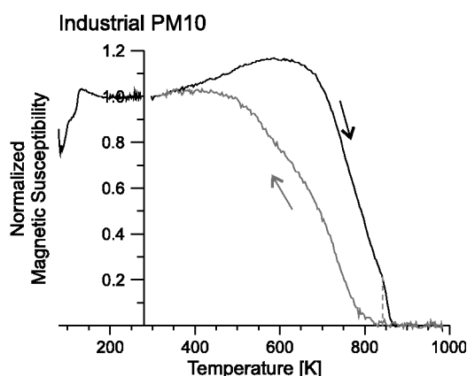
Teplovní závislost magnetické susceptibility vzorku polétavého prachu <10 mm (PM10) ze stanice Bartovice v průmyslové oblasti. Teploty Verweyova přechodu a Curieova bodu, typické pro hrubozrnný magnetit, jsou vyznačeny přerušovanými čarami.
