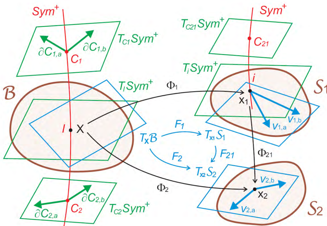
Schematické zobrazení vzájemných vztahů mezi veličinami popisující konečné deformace se zvýrazněním role prostoru deformačních tenzorů Sym^+
