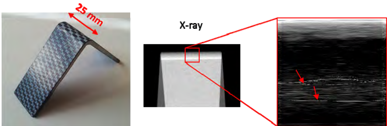
Detekce delaminace vrstev v ohybu uhlíkového kompozitu pomocí fázového efektu rentgenova záření. Zobrazení umožněné pomocí detektoru typu Medipix.
