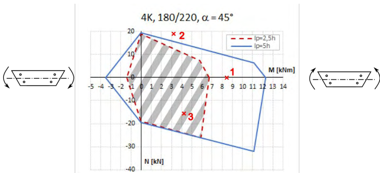
Návrhový diagram únosnosti navrženého spoje
