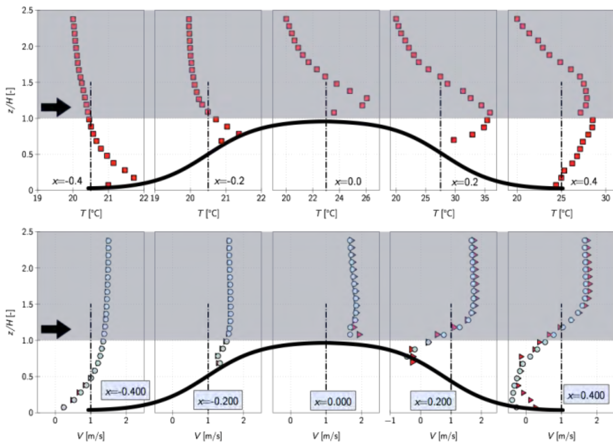
Výsledky modelování teploty horkého povrchu v závislosti na rychlosti větru a teplotních profilech
