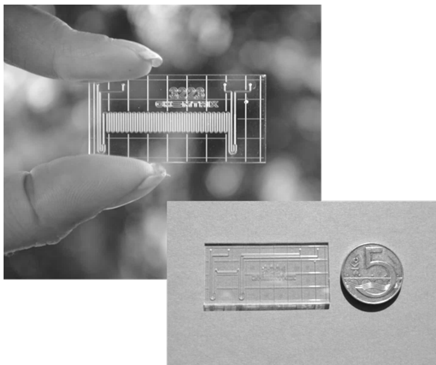
Mikrofluidní reaktory z křemenného skla testované pro stereoselektivní hydrogenace (horní o celkovém objemu 10 \mu\text{l} , spodní o objemu 1 \mu\text{l} )
