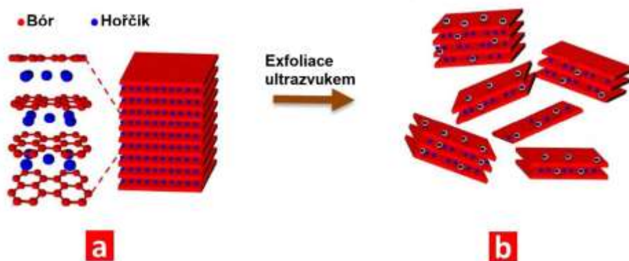
Vrstevnatá struktura diboridu \text{MgB}_2 (a)
