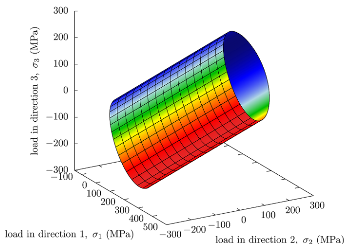
Obr. 3. Deformovaná plocha plasticity vymezující dovolenou oblast provozování konstrukce
