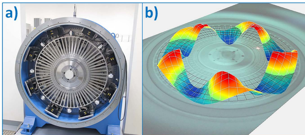
Obr. 2. a) Modelové turbínové kolo pro dynamickou kalibraci bezkontaktních senzorů vibrací rotujících lopatek b) Naměřené vibrace modelového lopatkovaného turbínového kola s 5 uzlovými průměry vybuzečné při 500 ot/min
