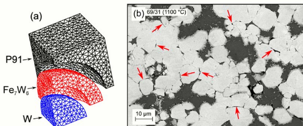
Obr. 4. a) konečně-prvkový model vícefázového kompozitu wolfram/ocel; b) reálná mikrostruktura kompozitu s viditelnými oblastmi nedokonalého propojení wolframových zrn (červené šipky)
