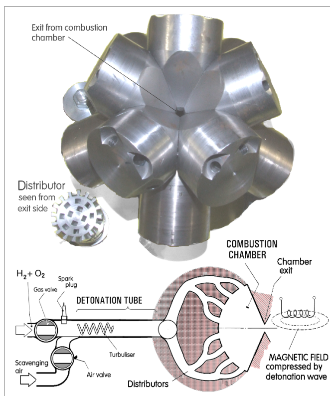
Obr. 1. Implozivní magnetokumulativní generátor
