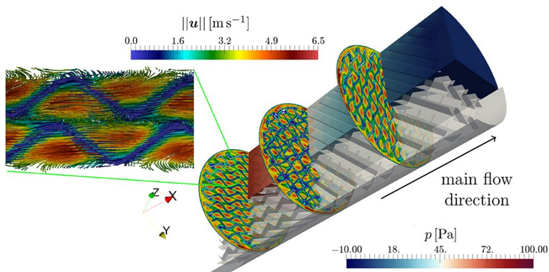
Obr. 11. Tlaková a proudová pole uvnitř separační kolony
