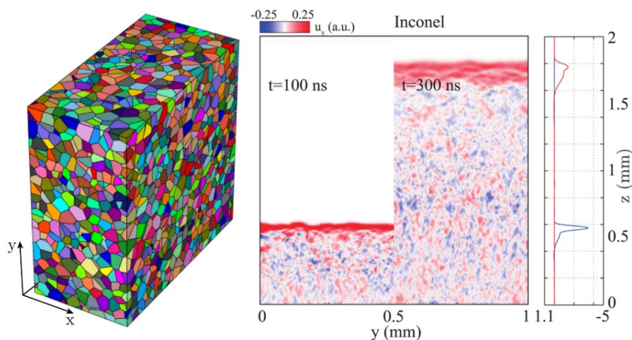
Obr. 9. Numerický model polykrystalu slitiny Inconel vytvořený Voronoiovou teselací a čítající 8000 zrn (vlevo) a simulace šíření ultrazvukových vln takovým prostředím (vpravo)
