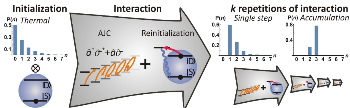
Obr. 3: Princip vybuzení a akumulace nekласičnosti pohybového stavu laserem zchlazeného iontu
