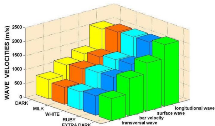
Obr. 13. Rychlosti napěťových vln v testovaných čokoládách.
