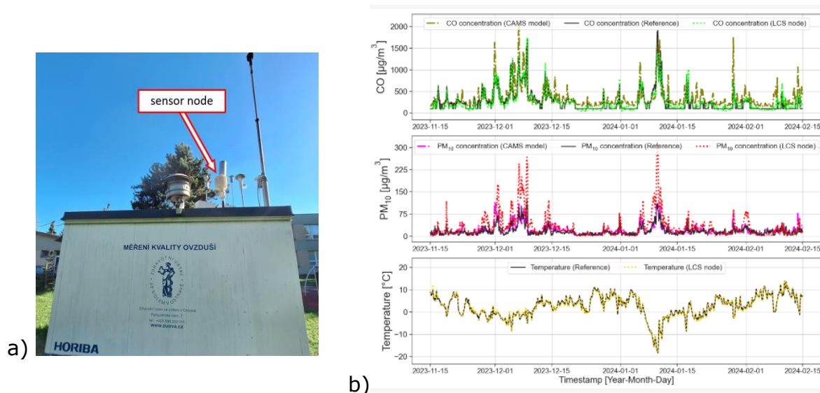
Obr. 11. a) Nízkonákladový senzorový uzel umístěný na střeše referenční stanice monitorování kvality ovzduší zdravotnického ústavu v Ostravě. b) výsledky porovnání vybraných hodinových datových řad ze zimního vyhodnocovacího období mezi CAMS modelem, referenčním měřením a novým „low-cost“ senzorem.
