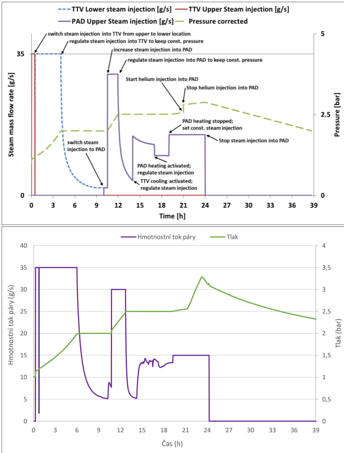
Obrázek 20: Časový průběh hmotnostního toku vstřikované páry a tlaku v systému. Srovnání očekávaných výsledků společností Becker Technologies (nahore) a výsledků simulace na SÚRO v.v.i. (dole)
