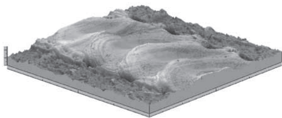
■ Simulace natavené stopy pomocí software TALYMAP a detail nataveného povrchu stopy o šířce 1,2 mm.
