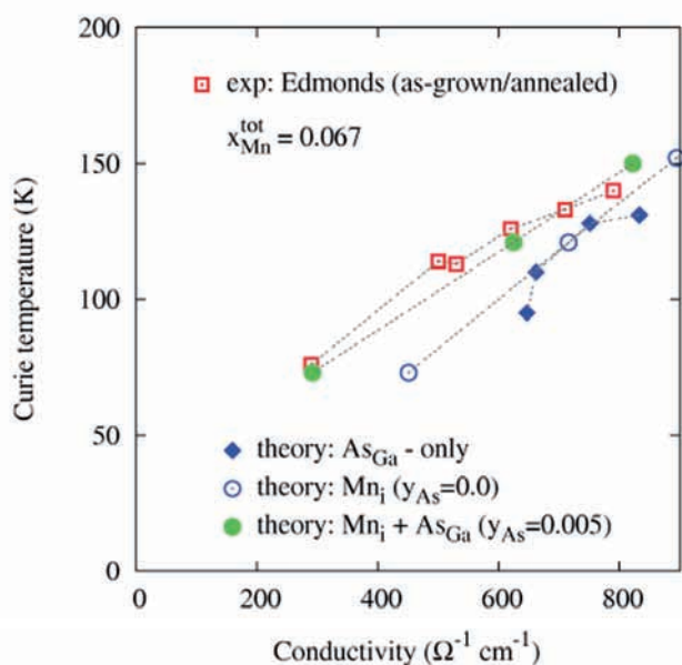
■ Srovnání teorie (zelené symboly) a experimentu (červené symboly).
