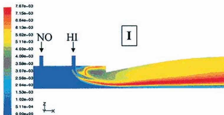
■ Kontury molárních frakcí chemicky generovaného atomárního jódu pro COIL.
