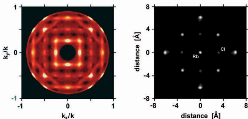
■ Hologram chloridu rubidného získaný z rozdílů difúzního rozptylu rentgenového záření naměřeného při energiích 15,060 keV a 15,120 keV (vlevo). Zrekonstruovaný reálný obraz atomů rubidia a chlóru v krystalografické rovině (001) (vpravo).
