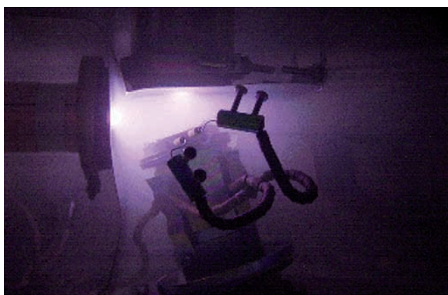
■ Systém s dvojitou dutou katodou během depozice vrstev \text{Ba}_x\text{Sr}_{1-x}\text{TiO}_3
