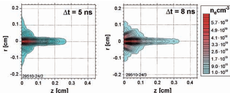
■ Podélný řez plazmovým jetem zformovaným na stříbrném terčíku při energii dopadajícího laserového svazku 100 J a poloměru ohniskové skvrny 300 \mu\text{m} v čase 5 ns (vlevo) a 8 ns (vpravo) po vzniku jetu. Vrstevnice byly získány pomocí laserové interferometrie a odpovídají různým hodnotám hustoty plazmatu. Na periférii jetu je elektronová hustota 1 \times 10^{18} \text{ cm}^{-3} .
