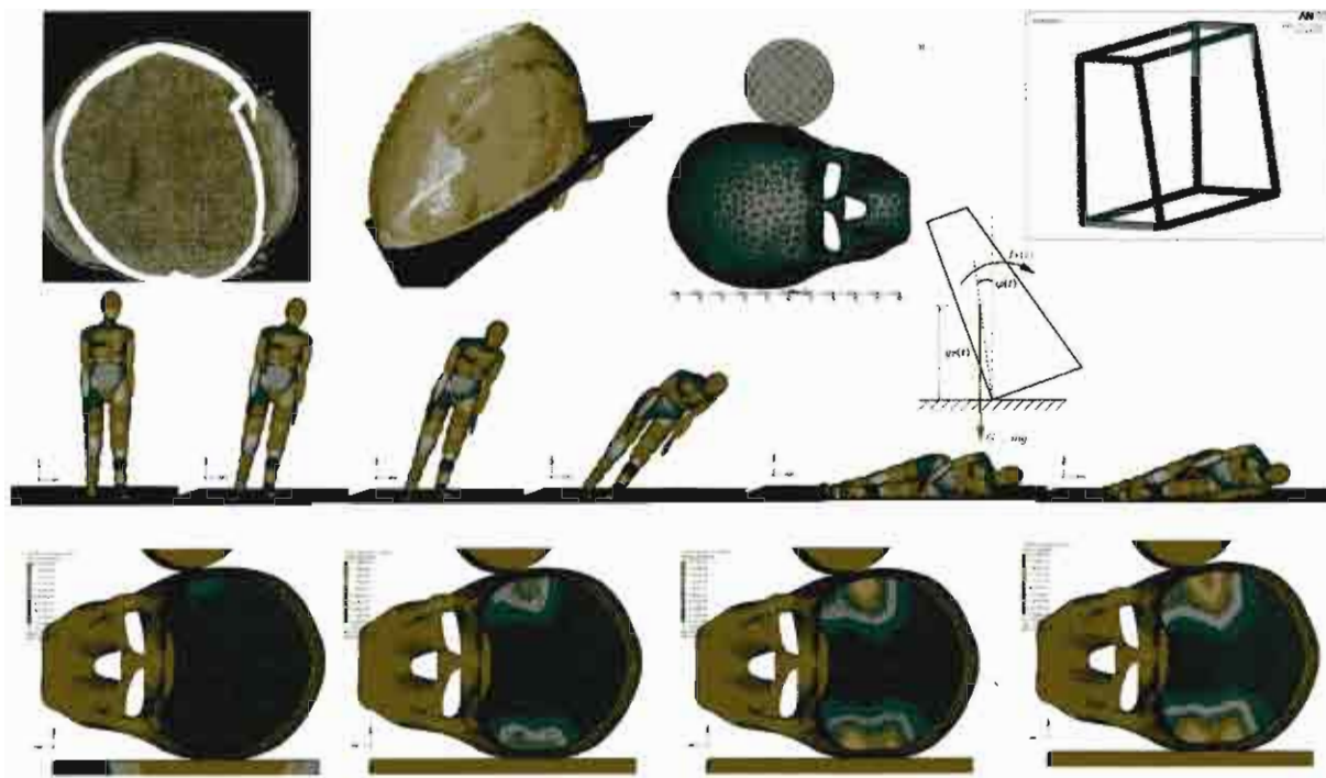
Modelová rekonstrukce sportovního úrazu hlavy
