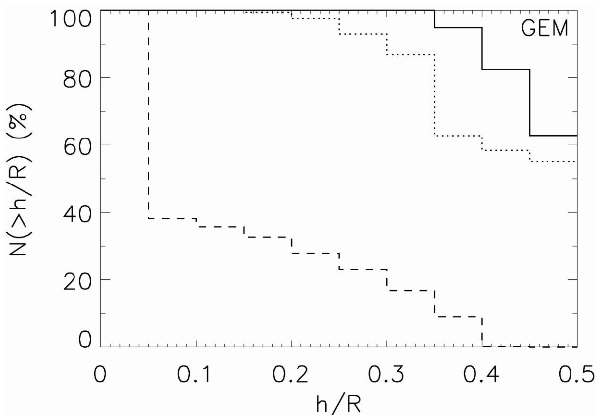
Obr. 4: Kumulativní četnost meteoroidů (v procentech) s hloubkou rozpuhané povrchové vrstvy větší než h/R (hloubka škálovaná poloměrem tělesa) pro roj Geminidy. Plná čára odpovídá tělesům o velikosti 10 cm, tečkovaná 1 cm a čárkovaná tělesům o velikosti 1 mm.
