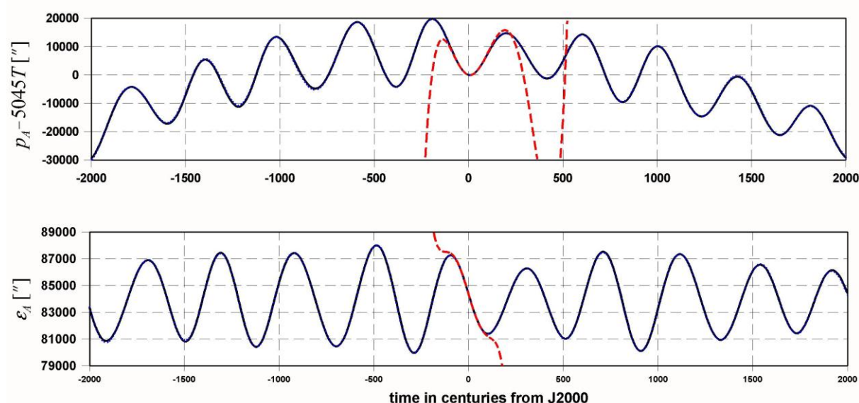
Obr. 5: Porovnání nového modelu (plná čára) s numerickou integrací (tečkovaná čára) a modelem IAU 2006 (čárkovaná čára) pro obecnou precesi v délce p_A a sklon ekliptiky \varepsilon_A . První dvě křivky jsou graficky nerozlišitelné.
