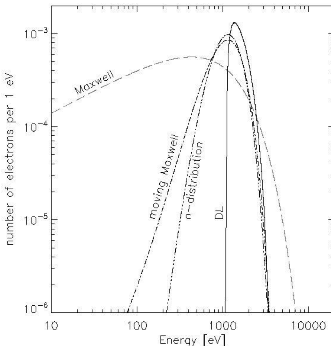
Obr. 4: Srovnání elektronových rozdělovacích funkcí se stejnou střední energií ve slunečních erupcích: n -rozdělovací funkce, pohybující se Maxwellova funkce a DL rozdělovací funkce, která vzniká ve dvojné vrstvě, jsou téměř stejné v jejich vysoko-energetické části. Klesají k vyšším energiím mnohem rychleji než Maxwellova rozdělovací funkce.
