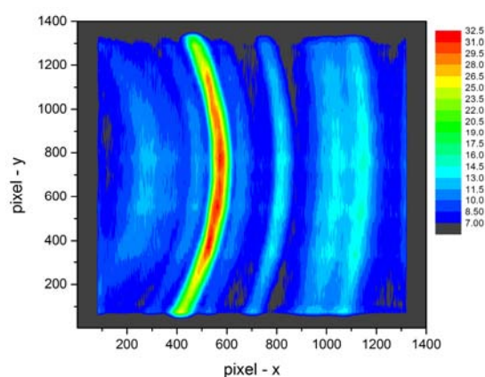
Obr. 5. Dvojdimenzionální detektor neutronů s vysokým rozlišením, vpravo ilustrační neutronový difraktogram.
