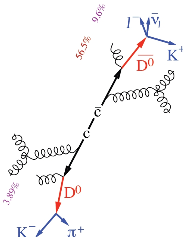
Produkce páru půvabného kvarku a antikvarku a zkoumané rozpady vzniklých D^0 mezonů.
