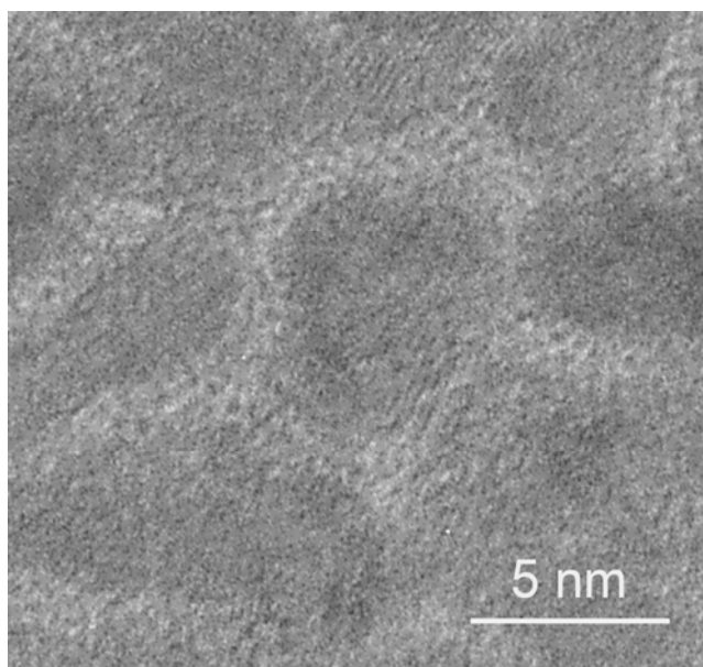
TEM snímek s vysokým rozlišením ukazující tvorbu nanokompozitní struktury Co-C 60 ve stavu po nanesení. Nanokompozitní struktura je výsledkem výrazné fázové separace v nanášené směsné vrstvě.
