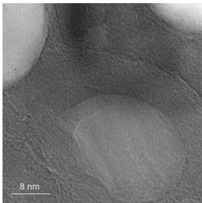
TEM snímek s vysokým rozlišením směsi Co-C 60 nanesené při pokojové teplotě (RT) s následným žíháním při teplotě 500°C po dobu 1 hodiny. Lze vidět vytvoření grafitického obalu okolo seskupení Co nanokrystalů.
