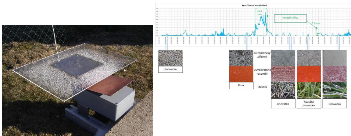
Obr.: Fotografie automatického rosoměru (a) a ukázka záznamu měření v březnu 2011 (b).
