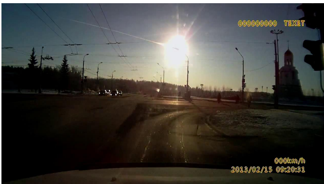
Obr. 1: Průlet planety zemskou atmosférou při pohledu z města Kamensk Uralskyj. (Autor snímku: Alexandr Ivanov.)
