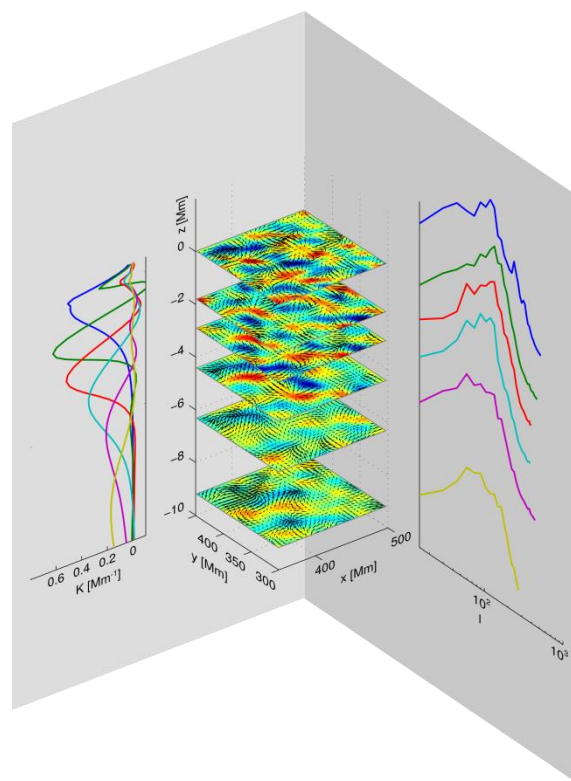
Obr. 5: Příklad struktury proudění na supergranulárních škálách v přívprchové vrstvě sluneční konvektivní zóny.
