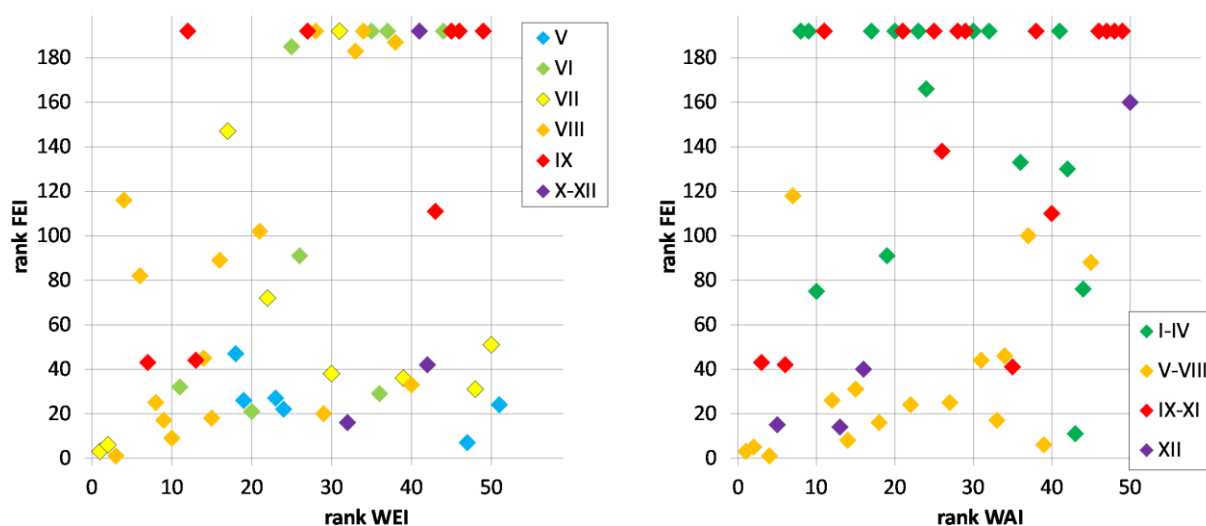
Obr. 8: Porovnání srážkových a povodňových událostí v ČR 1961-2010. Pořadí srážkových událostí podle jejich extremity (vlevo – WEI) a sezónní abnormality (vpravo – WAI) na ose x je porovnáváno s pořadím extremity případně následné povodně (FEI) na ose y. Případy bez větší hydrologické odezvy jsou koncentrovány v horních částech grafů.
