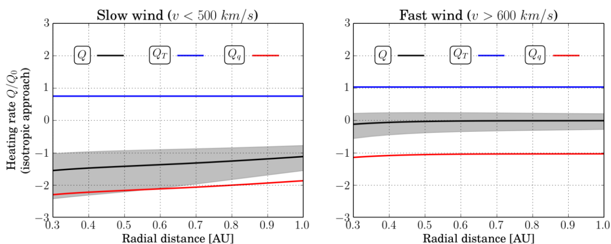
Obr. 3: Odhad normované energetické bilance elektronů ve slunečním větru jako funkce radiální vzdálenosti od slunce získaný z pozorování sond HELIOS 1/2. Míra ohřevu Q_T potřebná pro neadiabatickou expanzi (modrá čára) je kompenzována degradací elektronového tepelného toku Q_q (červená čára) představující záporný příspěvek k celkové energetické bilanci Q (černá čára). Vnitřní ohřev poskytovaný elektronovým teplotním tokem je dominantnější v pomalém slunečním větru (levý panel) než v rychlém slunečním větru (pravý panel). Šedá oblast znázorňuje konfidenční interval pro celkovou energetickou bilanci vyplývající ze statistických chyb v měření.
