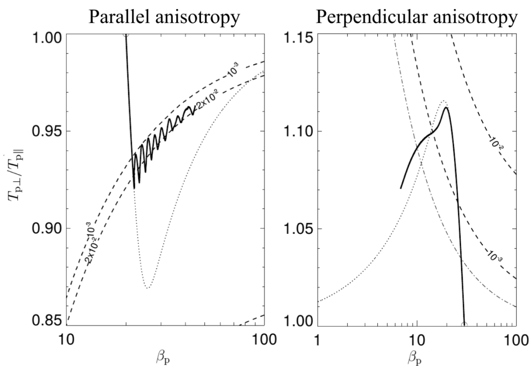
Obr. 16: Simulovaný vývoj protonové teplotní anizotropie (plná čára) je zobrazen jako funkce poměru kinetického a magnetického tlaku ( \beta_p ). Kontury maximálních růstových faktorů šikmé hadicové nestability pro paralelní teplotní anizotropii (levý panel) a zrcadlová nestability pro kolmou teplotní anizotropii (pravý panel) jsou znázorněny čárkovanou čarou. Tečkovaná čára pak ukazuje teoretický vývoj systému za přítomnosti pouze Coulombovských srážek.
