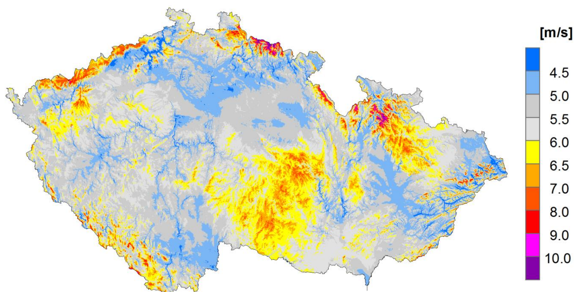
Obr. 4: Mapa zobrazuje průměrnou rychlost větru nad územím ČR ve výšce 100 m nad povrchem podle modelu VAS/WAsP. Tento model má ve výsledné větrné mapě váhu 70 %, zbývajících 30 % reprezentuje model PIAP.
