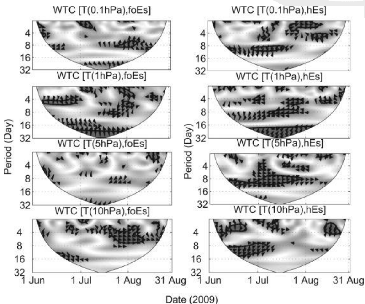
Obr. 12: Waveletová koherence mezi teplotami na čtyřech tlakových hladinách v stratosféře a dolní mezosféře a kritickou frekvencí sporadické vrstvy E foEs (levé panely) a její výškou hEs (pravé panely) pro srpen 2009.
