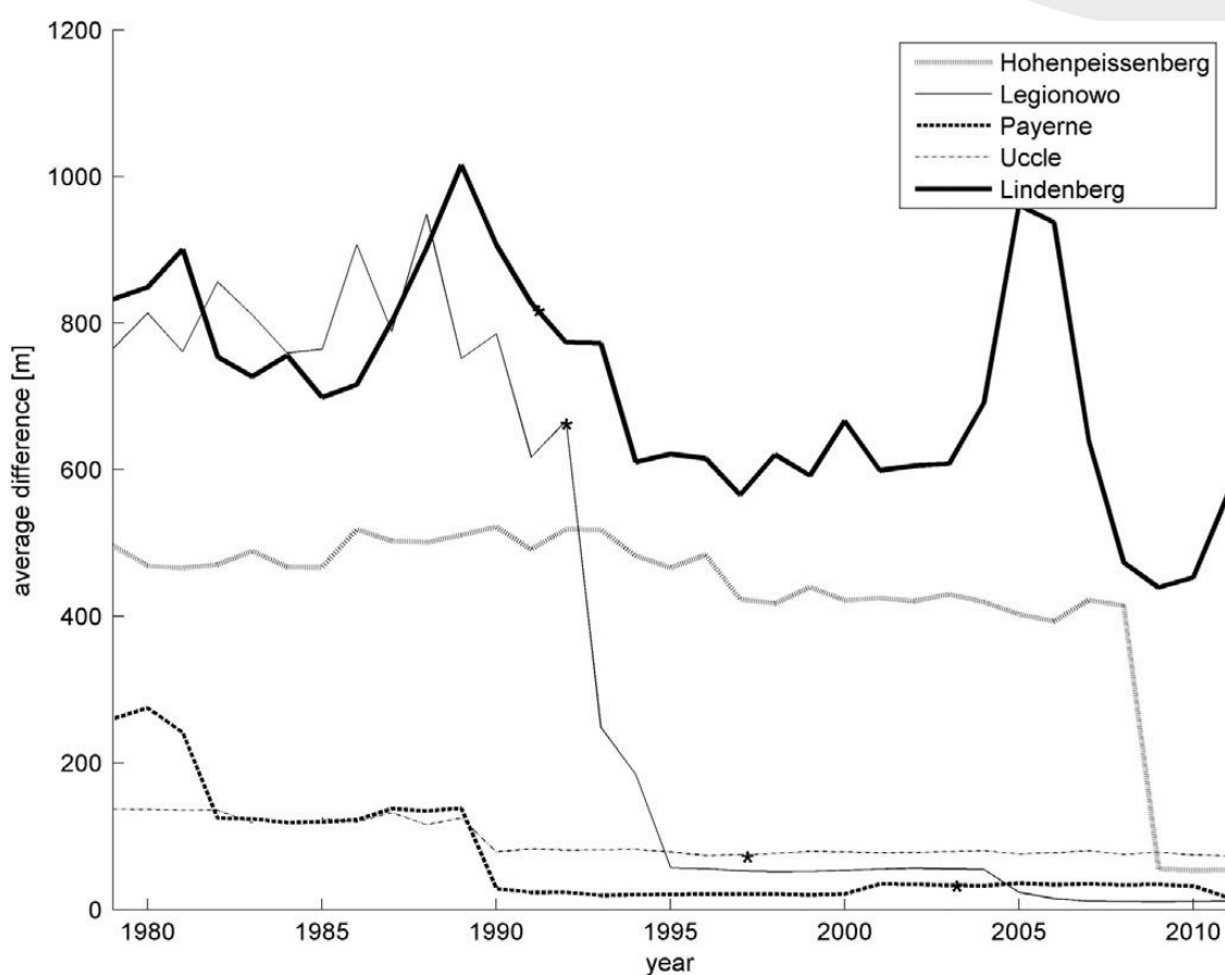
Obr. 17: Vývoj vertikálního rozlišení měření evropských ozonosondážních stanic. Hvězdičky označují, kdy došlo ke změnám typu ozónových sond.
