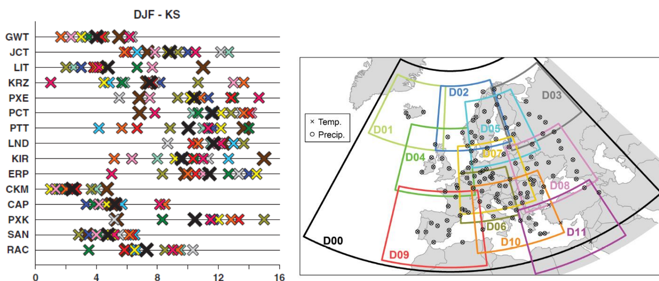
Obr. 13: Pořadí klasifikačních metod (řádky) podle jejich schopnosti charakterizovat přízemní teplotu a srážky, kvantifikované kritériem založeným na Kolmogorovově-Smirnovově testu, v němž pro jednotlivé oblasti (odlišené barvou křížků; umístění oblastí je na obrázku vpravo). Velký černý křížek označuje průměrné pořadí. Metody s převládajícím nízkým pořadím (např. GWT – podobnost s cirkulačními prototypy, LIT – Litynského metoda, CKM – shluková analýza pomocí algoritmu k-means, SAN – SANDRA) jsou k popisu přízemních klimatických proměnných vhodnější.
