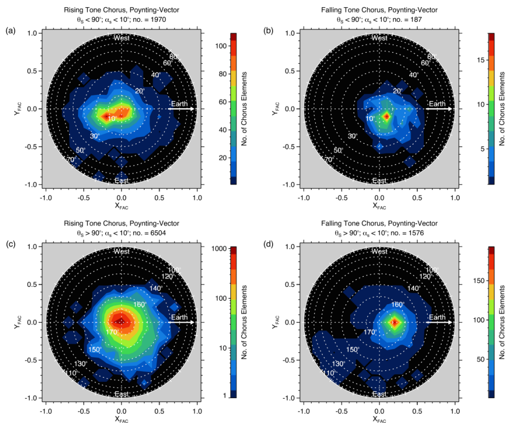
Obr. 9a: Směr Pyntingova vektoru v ploše [x, y] v souřadném systému magnetického pole Země. Levé panely zobrazují vlastnosti stoupavých tónů emise chorus, pravé panely vlastnosti klesajících tónů. Barevná škála znázorňuje počet případů vstupujících do statistiky.
