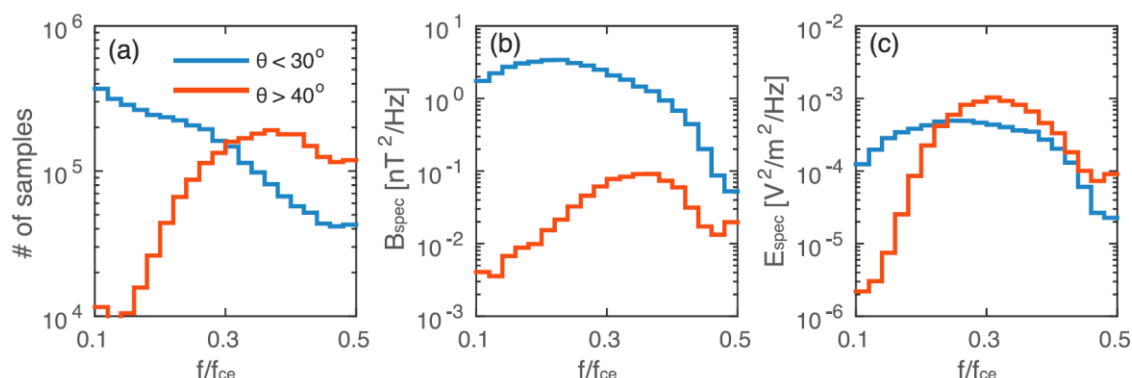
Obr. 9b: Vlastnosti kvaziparalelního (modré křivky) a kvazielektrostatického (oranžové křivky) módu spodního pásu elektromagnetické emise typu chorus (počet spektr vstupujících do analýzy (a), spektrální výkonová hustota magnetického (b) a elektrického (c) pole jako funkce frekvence normalizované elektronovou cyklotronovou frekvencí.
