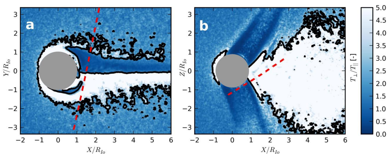
Obr. 11: Teplotní anizotropie iontů v okolí Jupiterova měsíce Io. Rozložení iontové teplotní anizotropie v okolí měsíce Io získaná z hybridní simulace interakce měsíce s okolním plazmatem. Panely ukazují teplotní anizotropii ve dvou rovinách, kolmé (vlevo) a podélné (vpravo) vzhledem k pozadovému magnetickému poli. Červená čára ukazuje průběh trajektorie sondy Galileo do obou rovin. Černá čára ohraničuje oblast očekávaného výskytu iontových cyklotronových vln. Ve shodě s lokálními měřeními se tato oblast nachází převážně za měsícem po směru toku okolního plazmatu.
