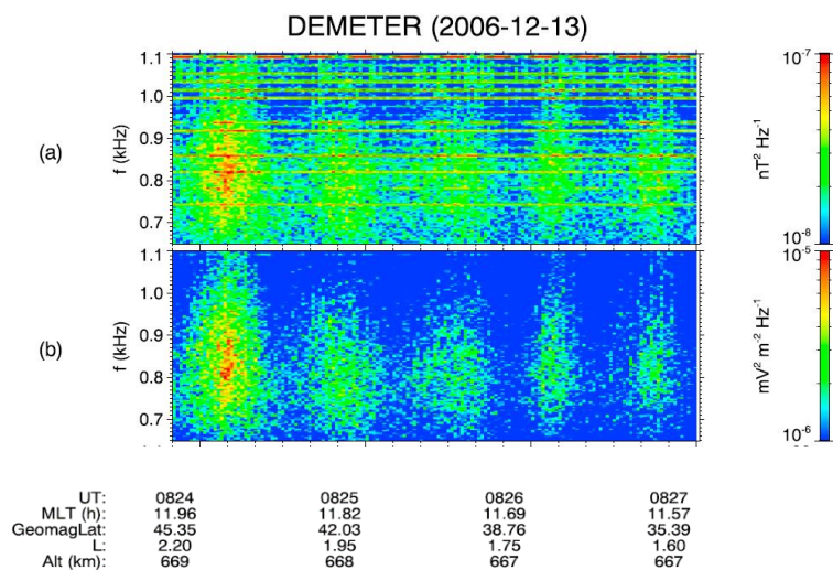
Obr. 14a: Příklad kvaziperiodické emise zaznamenané družicí DEMETER.
