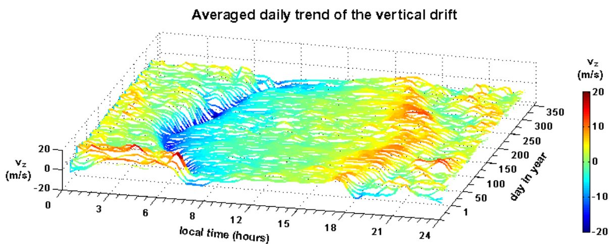
Obr. 15: Změny denního průběhu vertikálních driftů během roku. Vliv východu a západu slunce je jasně patrný; pravidelné chování během dne a nepravidelné v noci.
