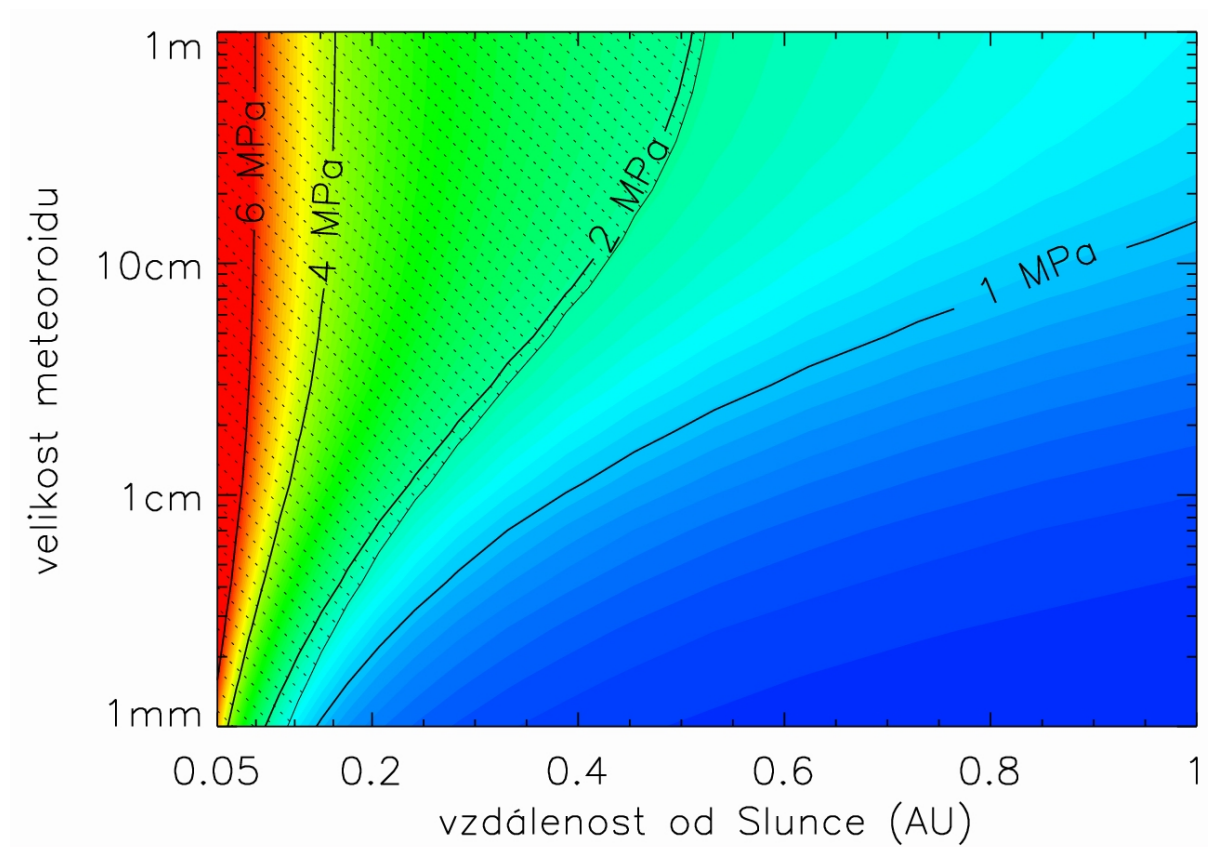
Obr. 3: Tepelné napětí v centru meteoroidu v závislosti na vzdálenosti od Slunce (osa x) a velikosti meteoroidu (osa y). Izobary jsou označeny hodnotou napětí v megapaskalech. Šrafovaně je znázorněna oblast, ve které tepelné napětí překračuje pevnost materiálu meteoroidu. Předpokládá se, že rotační osa meteoroidu je kolmá vůči směru ke Slunci a složení odpovídá uhlíkatým chondritům. Rotační perioda P je svázána s velikostí tělesa D vztahem: P(s)=3/D(m) .
