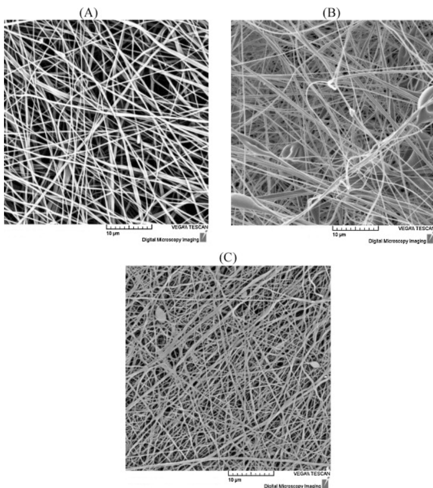
SEM mikrofotografie nanovláknenných membrán připravených z polystyrenu (A), polyfenylenoxidu (B) a polyurethanu (C)
