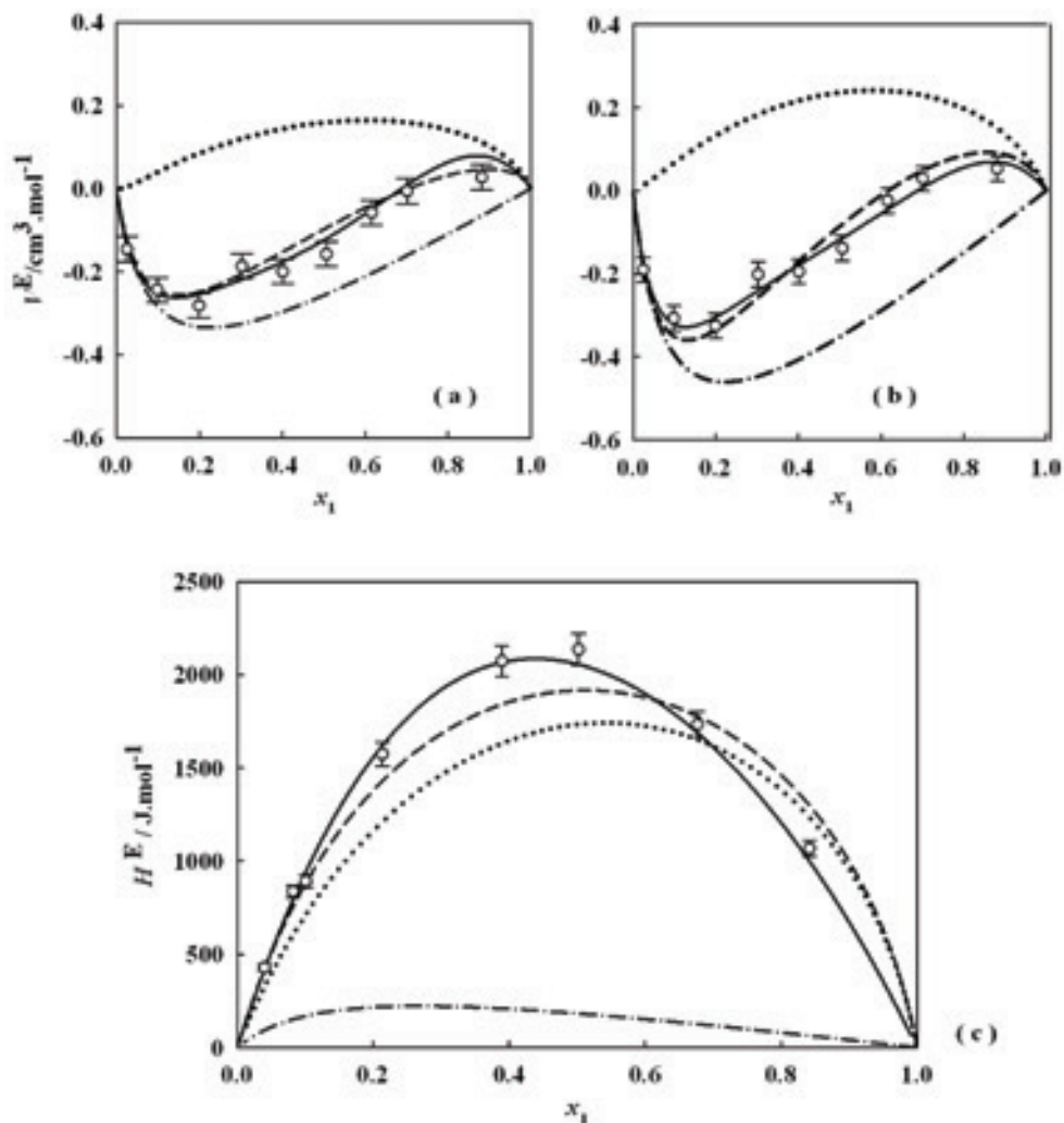
Dodatkový objem ( V^E ) v závislosti na složení při 298.15 K (a) 303.15 K (b) dodatková entalpie ( H^E ) v závislosti na složení při 303.15 K (c) v systému [\text{N}_{6,222}][\text{Tf}_2\text{N}] + \text{methanol} . Experimentální data a modelovaný průběh závislostí Redlichovou-Kisterovou rovnicí a modelem ERAS
