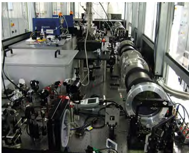
■ Obr. 7 Výkonová část 10 J / 10 Hz laserového systému pro řetězec L2, testovaný v laboratoři FZÚ Sofia. Systém využívá kryogenní multideskový zesilovač vyvinutý STFC Rutherford Appleton Laboratory (Velká Británie), zbytek systému včetně oscilátoru, čela laserového řetězce a kryogenní chladicí jednotky (teplota cca 150 K) byl navržen a vybudován pracovníky oddělení 91.
