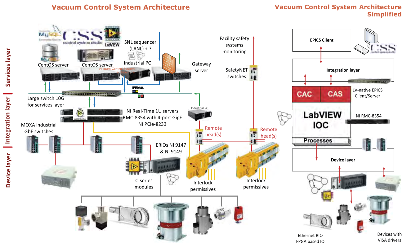
Obr. 4 Architektura řídicího a zabezpečovacího systému vakuového kompresoru pulsů laserového systému L1. Relativní složitost systému, který využívá komerčně dostupné komponenty, je dána mimo jiné potřebou plné automatizace provozu laseru, vysokým průměrným výkonem (100 mJ/1 kHz) a potřebou přístrojové ochrany v případě selhání některé komponenty.
