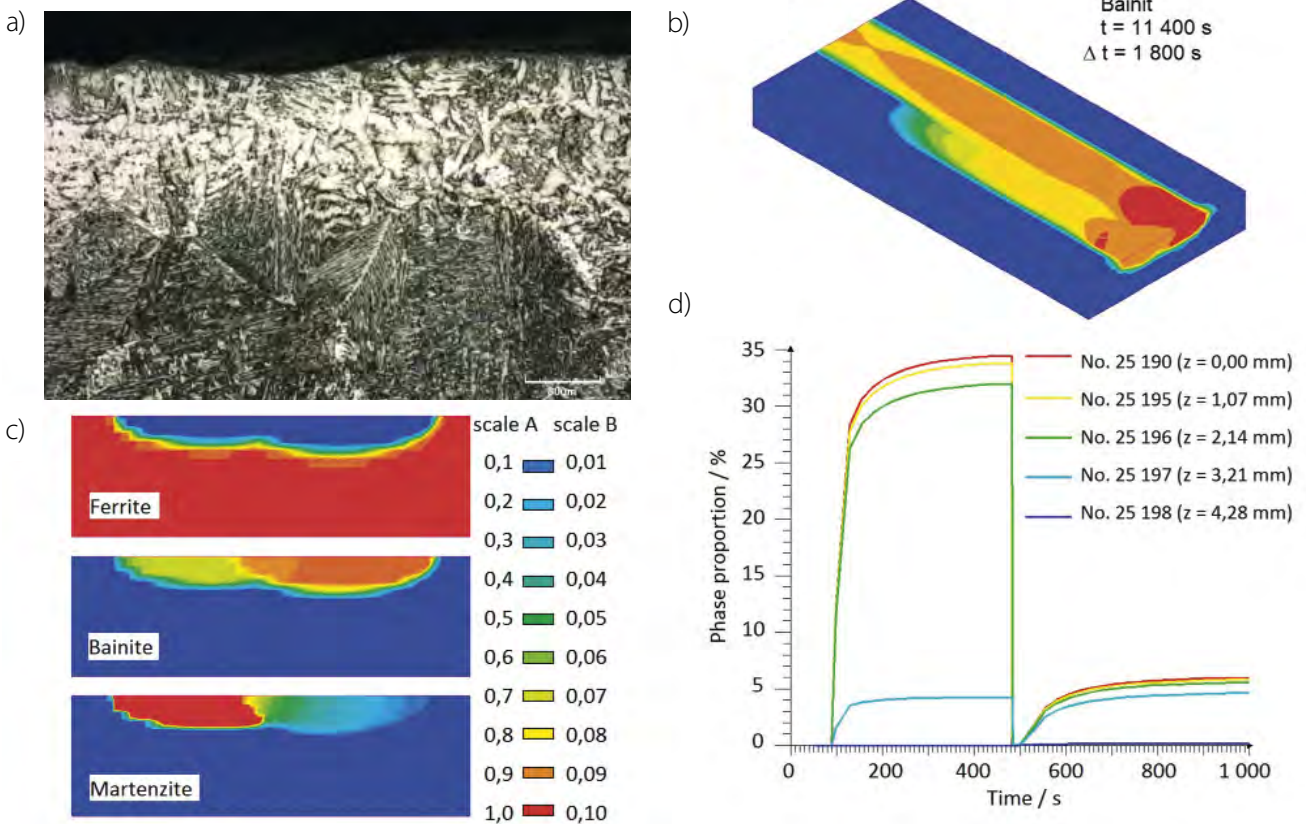
■ Obr. 1 Příčný řez oblastí překryvu stop laserem přetaveného povrchu oceli S355JR (a), 3D model zastoupení bainitu při časovém odstupu aplikace laseru 1 800 s (b), 2D model konečného rozložení metalografických fází (c), časový vývoj zastoupení martenzitu v ose překryvu přetavených stop (d).
