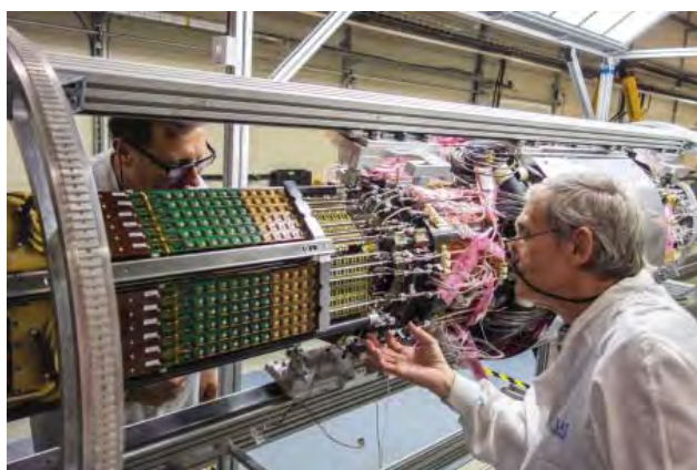
Obr. 1 Pracovník Fyzikálního ústavu Michal Tomášek při modernizaci pixelového detektoru experimentu ATLAS.
