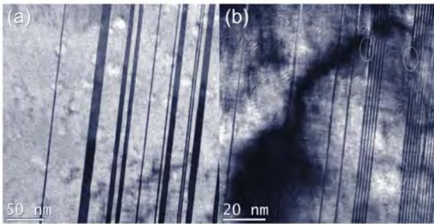
■ Obr. 12 Směs nemodulované a zdvojitěné 14M fáze na nanoúrovni. (a) Zbytková 14M fáze (tmavé proužky) v nově formované fázi nemodulované. (b) Kontrast ukazující jednotlivá nanodvojčata. Kroužkem jsou označena místa mizejících dvouvrstevných dvojčat.
