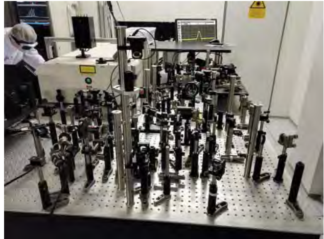
■ Obr. 11 Vývojový systém generátoru ultra širokopásmového koherentního laserového zdroje, tzv. White Light, v laboratoři FZÚ Sofia. Generátor je vyvíjen pro přídavný (sondovací) svazek systému L2 na vlnové délce 2,2 \mu\text{m} .
