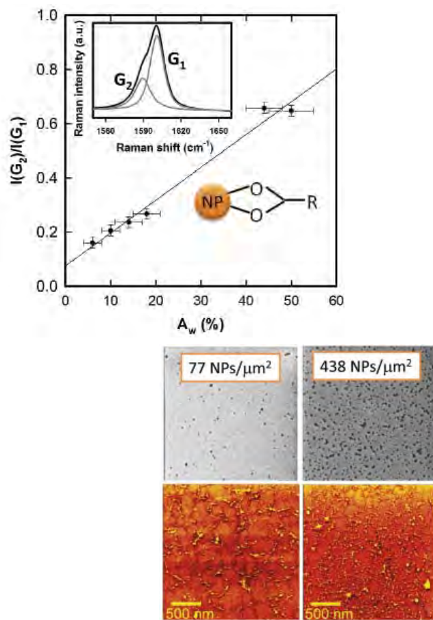
■ Obr. 7 Obecná korelace mezi zvrásněnou frakcí grafenu ( A_w ) a relativní intenzitou stěžejního Ramanského aktivního módu grafenu ( G ) příslušejícího zvrásněné vrstvě (vlevo). V detailu je znázorněn rozklad spektra G módu na zvrásněnou ( G_2 ) a hladkou ( G_1 ) frakci. Vpravo je uvedeno srovnání topografie substrátu dekorovaného magnetickými nanočásticemi (šedé obrázky) a výsledné zvrásněné monovrstvy grafenu pro dvě různé koncentrace nanočástic (barevné obrázky).
