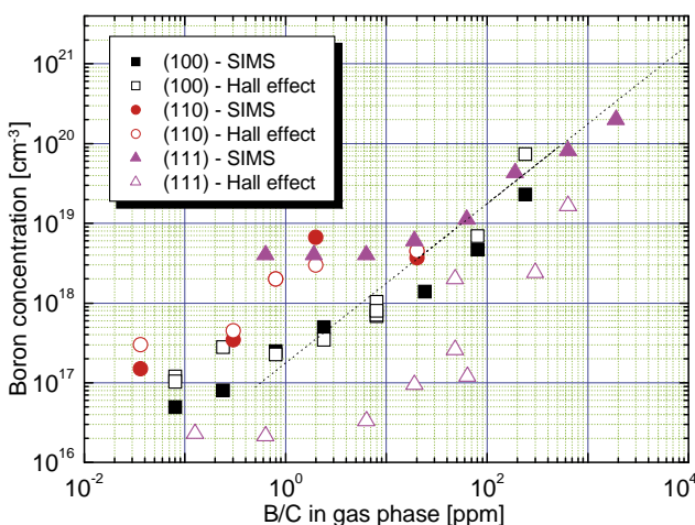
■ Obr. 17 Celková koncentrace bóru obdržena pomocí SIMS a koncentrace akceptorů získaná z měření Hallova efektu na narostlých epitaxních diamantových vrstevách na orientaci substrátu (100) a (111) vynesena v grafu jako funkce poměru B/C v plynné směsi.
