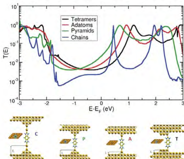
■ Obr. 13 Vypočtená transmisní spektra molekulárních obvodů založených na karbenu připojeném ke zlatému povrchu přes různé struktury hrotu: tetramer (T), adatom (A), pyramida (P) a řetězovitá struktura (C).
