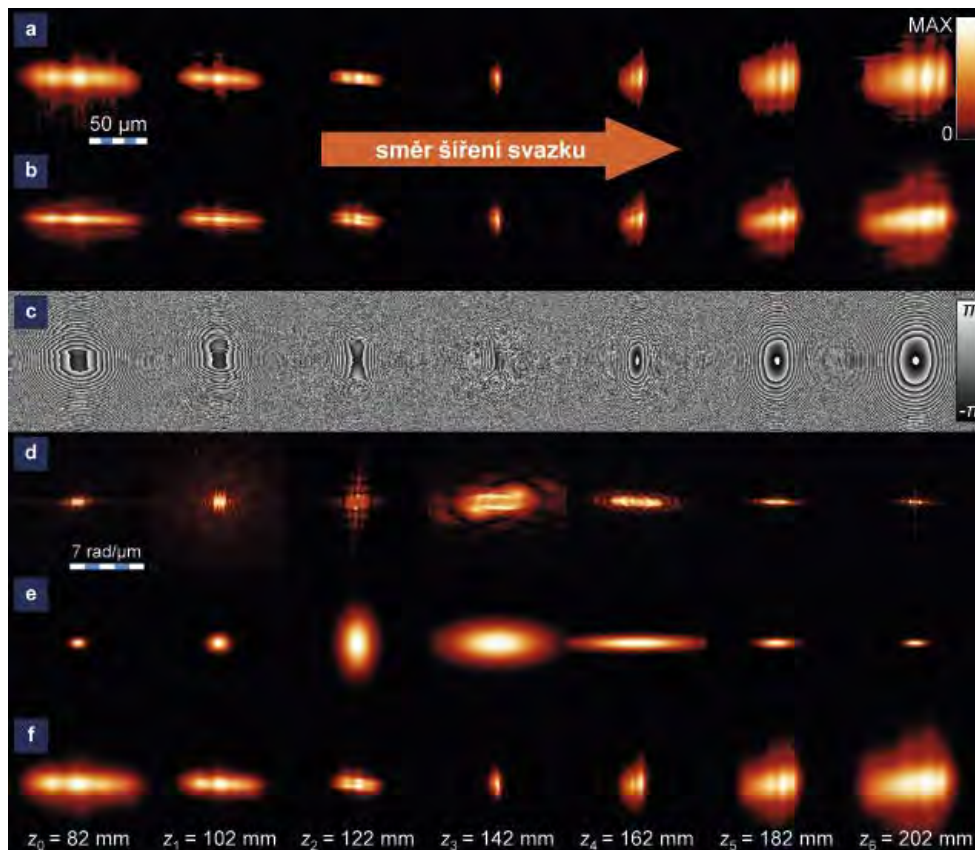
■ Obr. 14 Výstup fázově-rekonstrukčního kódu PhaRe [20]. (a) Změřené amplitudy elektrického pole, (b), (c) amplituda a fáze rekonstruovaného zcela koherentního pole, (d), (e) rekonstruovaná amplituda komplexního stupně koherence a fit astigmatického gaussovského Schellova modelu, (f) amplituda elektrického pole optimalizovaného na částečnou koherenci.
